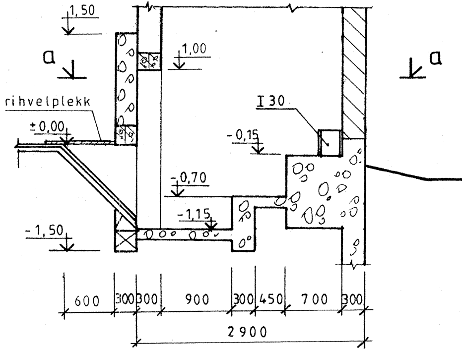
a - a M 1:50
