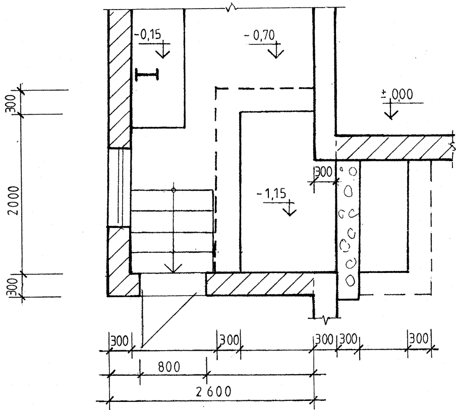
a - a M 1:50
